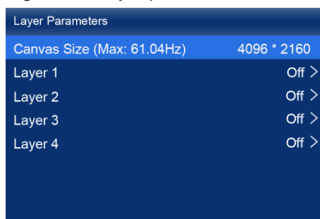
Figure 6-8 Layer parameters
