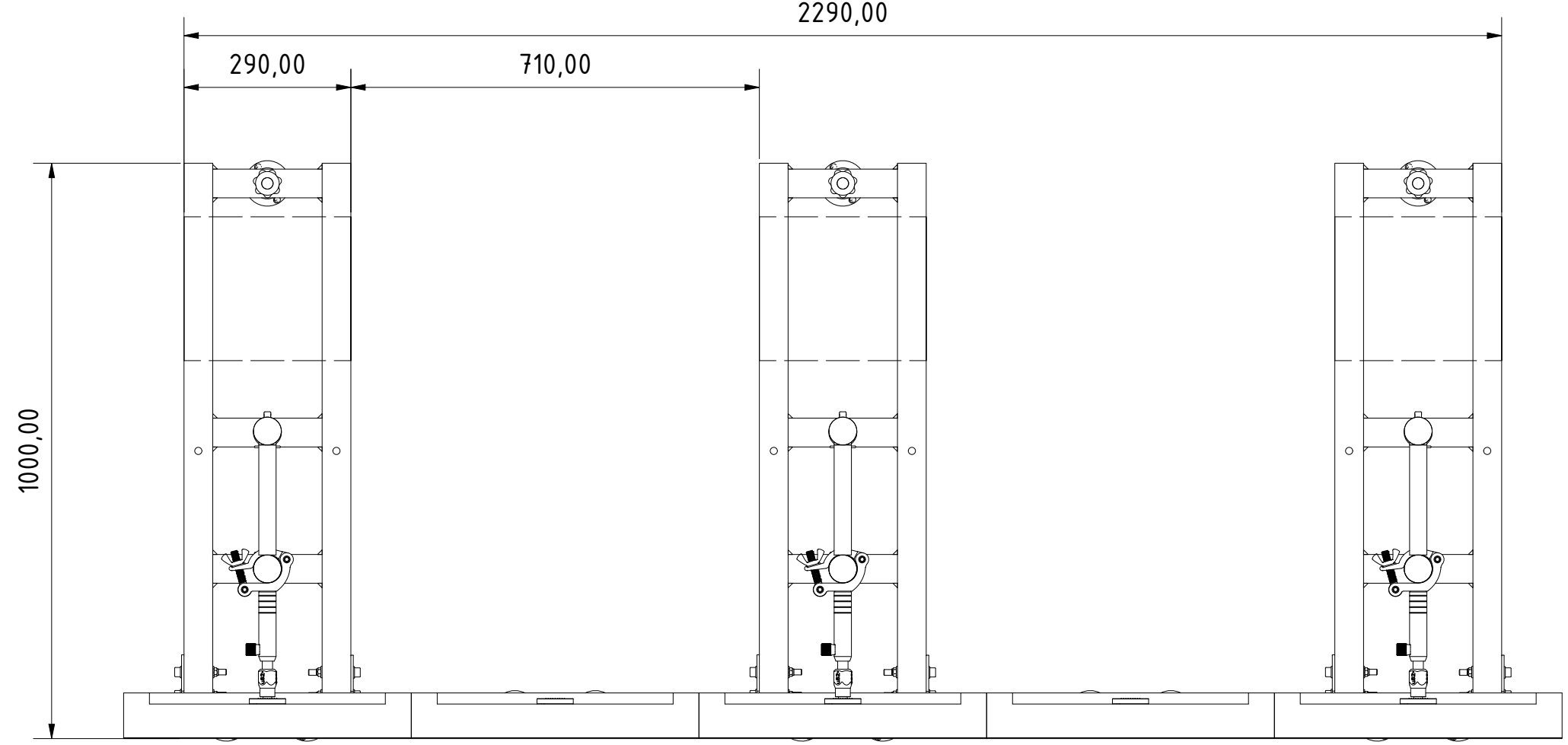
Draufsicht
