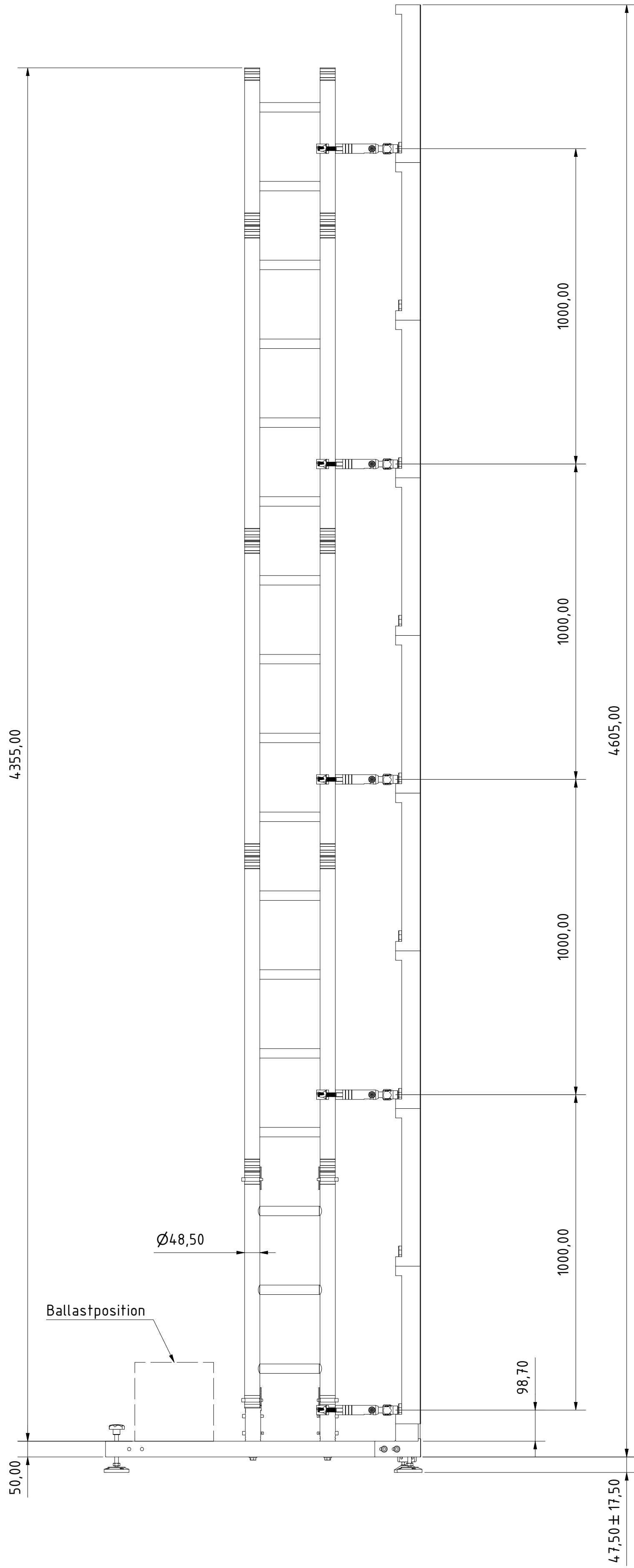
Seitenansicht
